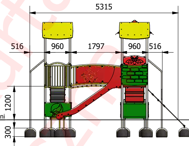
WIDOK 2
