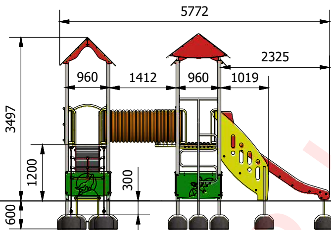
WIDOK 1
