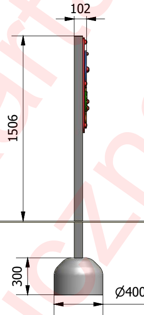
WIDOK 2
